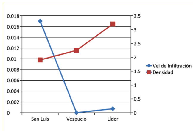
Figura N° 2. Comparación entre velocidad de infiltración (cm³/t) y densidad (g/cm³).
